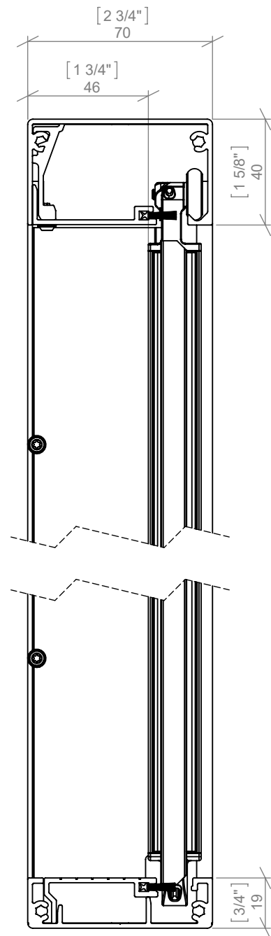
SECTION A-A
